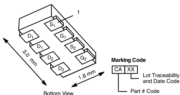
1206-8 ChipFET®
