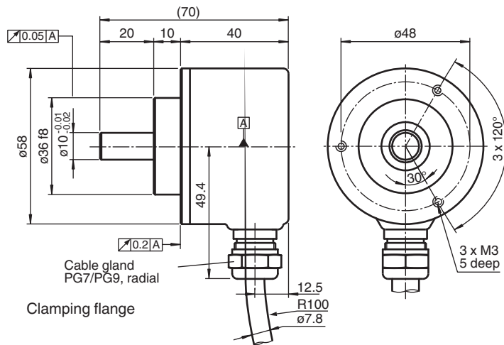
Servo flange
