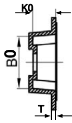
A0-A0
