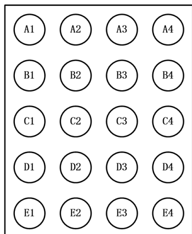
TPT24857-WS8R WLCSP20
